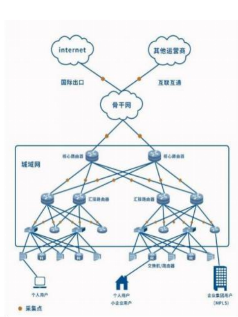
图2: 宽带骨干网
