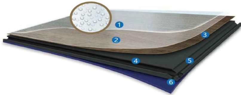
SPC地板产品结构图
