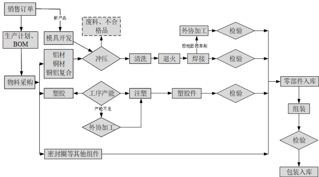
(2) 动力锂电池壳体的主要生产工艺及模式
