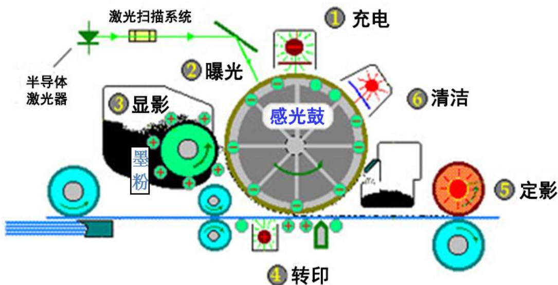
图：有机光导鼓静电成像过程
