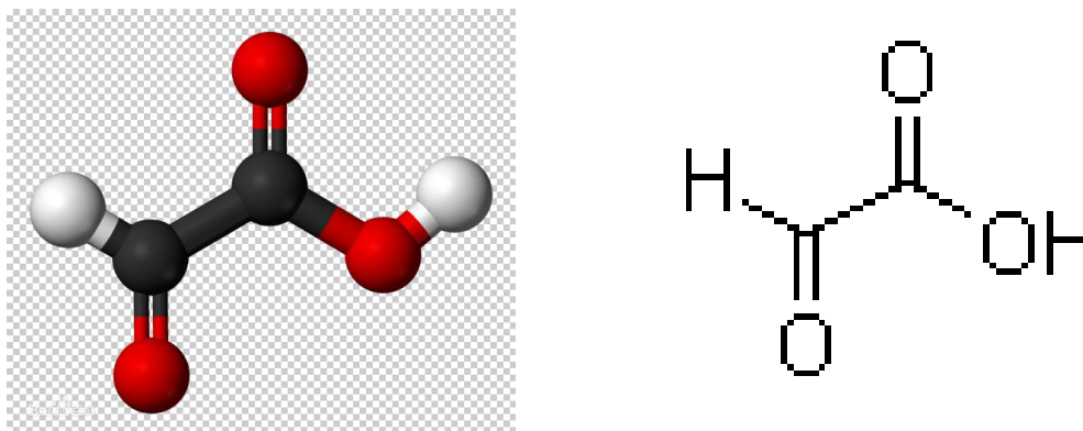
图：乙醛酸分子式
